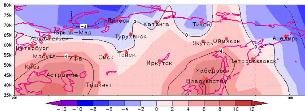
ФАКТИЧЕСКИЕ АНОМАЛИИ ПРИЗЕМНОЙ ТЕМПЕРАТУРЫ ВОЗДУХА ЗА НЕДЕЛЮ 05.12-11.18.24 Наблюдения (236 станций)
