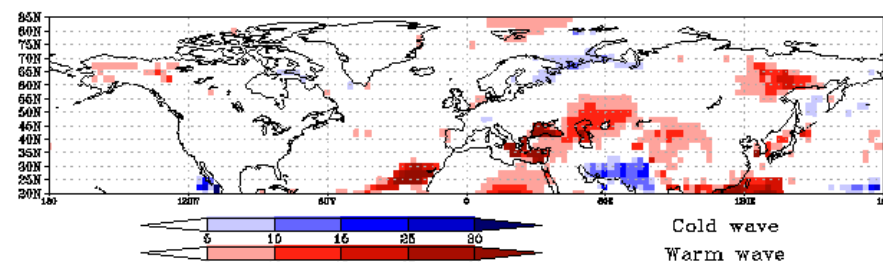
ПРОДОЛЖИТЕЛЬНОСТЬ ВОЛН ХОЛОДА (P<10%) И ТЕПЛА (P>90%) В ДНЯХ Прогноз на 46 суток от 18.04.24 (модель ПЛАВ)
