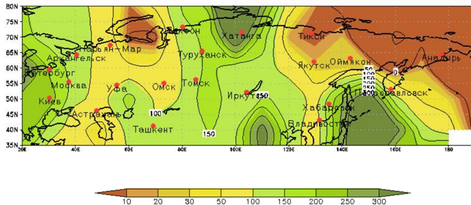
ФАКТИЧЕСКИЕ АНОМАЛИИ ОСАДКОВ (в % от нормы) 31.05-06.06.24 Наблюдения (236 станций)
