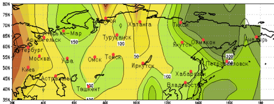
ФАКТИЧЕСКИЕ АНОМАЛИИ ОСАДКОВ (в % от нормы) 10.05-16.05.24 Наблюдения (236 станций)
