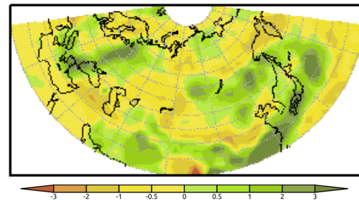
Модели Гидрометцентра России (SL-AV) и ГГО
