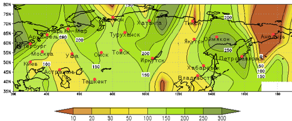
ФАКТИЧЕСКИЕ АНОМАЛИИ ОСАДКОВ (в % от нормы) 29.03.-04.04.24. Наблюдения (236 станций)
