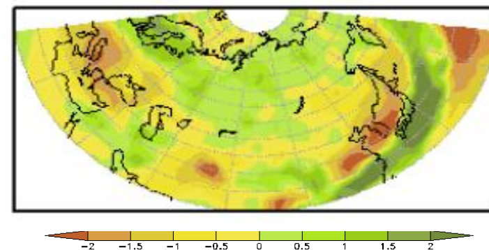
ПРОГНОЗ АНОМАЛИЙ ОСАДКОВ. Модели Гидрометцентра России (SL-AV) и ГГО. Прогноз на неделю 05.04-11.04.24.
