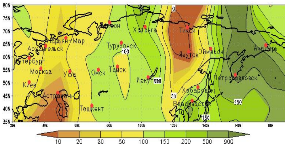
ФАКТИЧЕСКИЕ АНОМАЛИИ ОСАДКОВ (в % от нормы) 4-10.08.23. Наблюдения (236 станций)
