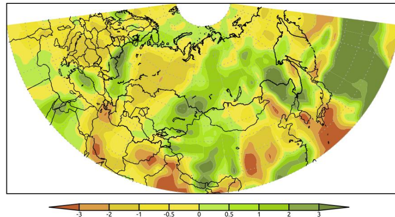
Прогноз аномалий количества осадков [мм/сут]. Модели: ГМЦ + ГГО Период прогноза: 11.08-17.08.2023, 1-я неделя
