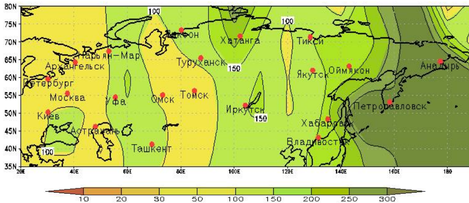
ФАКТИЧЕСКИЕ АНОМАЛИИ ОСАДКОВ (в % от нормы) 8.06.-6.07.23. Наблюдения (236 станций)
